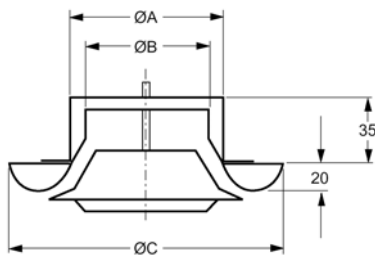
DVLI 80 – 125
