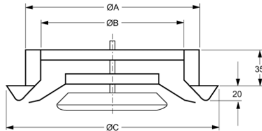
DVLI 160 – 200
